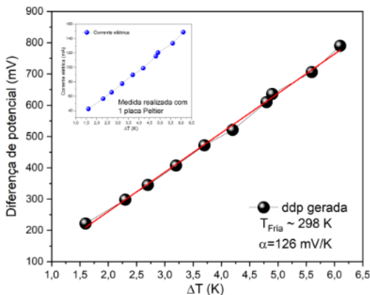
Gráfico 2: ddp em função da diferença de temperatura para placas Peltier.
