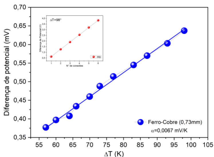
Gráfico 1: ddp em função da diferença de temperatura para fio de cobre de diâmetro 0,730mm
