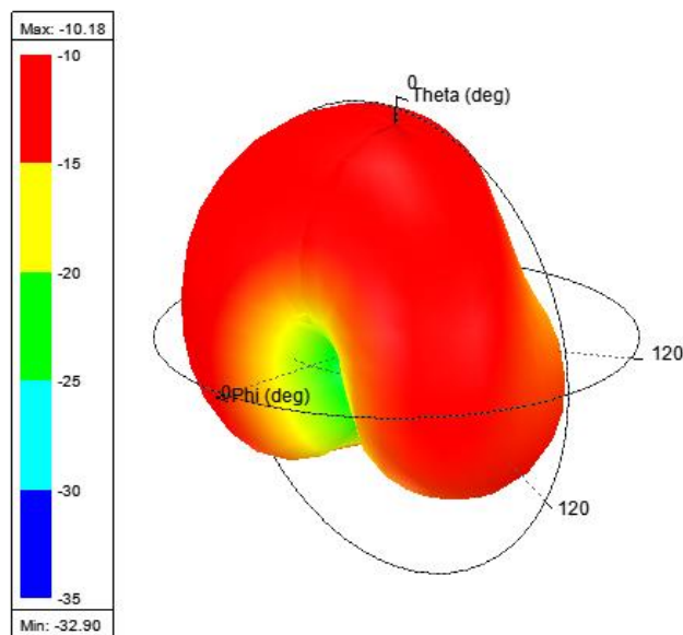
FIGURA 6. Diagrama de radiação 3D.
