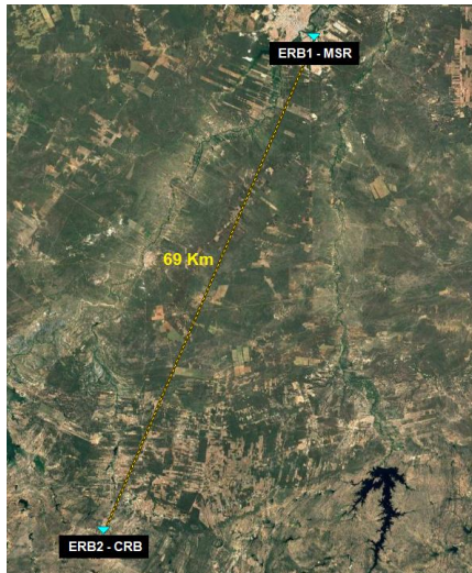
Fig. 4. Mapa com visada direta entre o campus leste da UFRSA Mossoró e o campus UFRSA Caraúbas.
